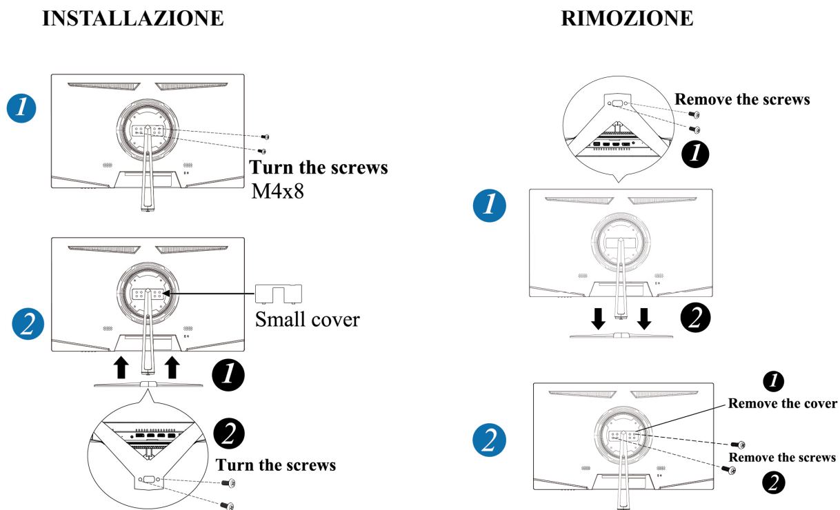
Figura.1. Installazione e Rimozione della Base
