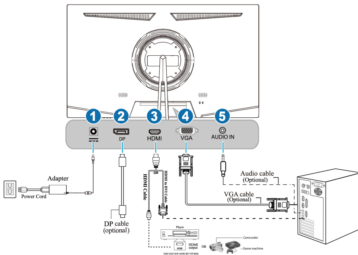
Figura 2. Collegamento al pc
